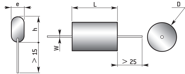
Sorties radiales Modèle PP 16 R
