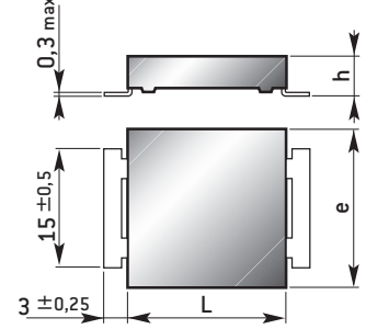
SMD leads / Sorties CMS : Models/Modèles PM 90 RT 2
