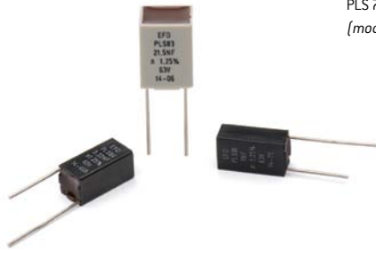
The outer foil is to the left of the marking L'armature extérieure est à gauche du marquage
