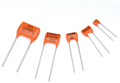
CM 04 to/à CM 08 CMR 03 to/à CMR 07
