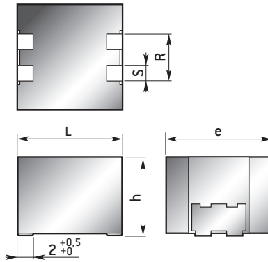
SMD leads / Sorties CMS : Models/Modèles PM 94 - PM 94 S
