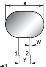
Sorties radiales Modèle PM 89 R enrobé
